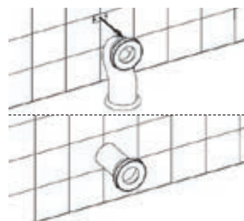
Vario odpad umožňujúci vodorovné alebo zvislé napojenie
