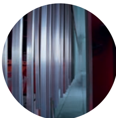
Lakovňa RAVAK Elektrostatické nanášanie práškovvej farby na hliníkové profily sprchových kútov, dverí a vaňových zásten.
